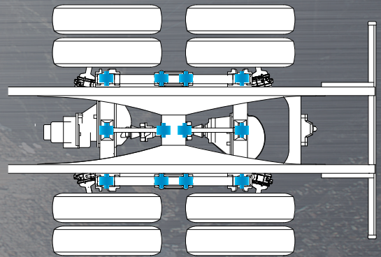
上面図
