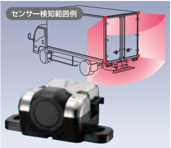
90 バックセンサー
