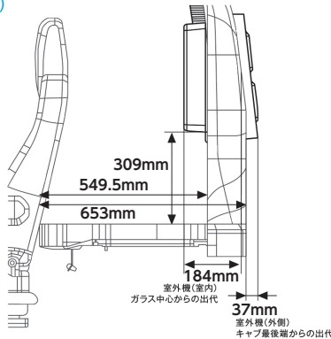
GIGAハイルーフ 装着レイアウト図 (室外機・側面)
