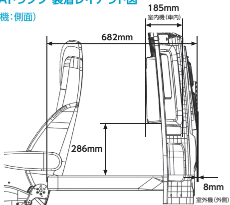
室外機(外側)
