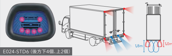
E024-STD6 (後方下4個、上2個)
