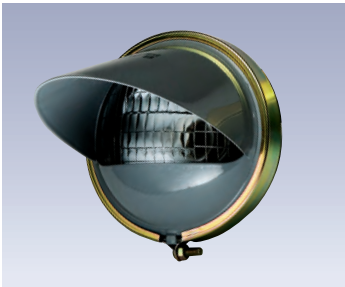
99 路肩灯 ●右側用/左側用 夜間時の安全走行に役立ちます。 ※架装仕様並びに取付位置等により取付時間は異なります。
