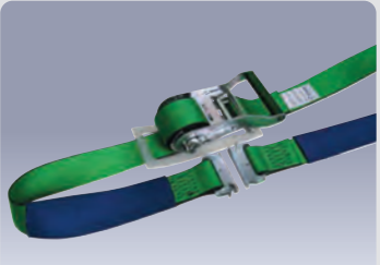
108 ラッシングベルト (ラチェット式) ●端末仕様：ナローフック&しぼり 全長6m (固定側1m/調整側5m) ●端末仕様：ワンピース 全長3m (固定側1m/調整側2m) 他各種設定
